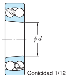
Agujero cónico
