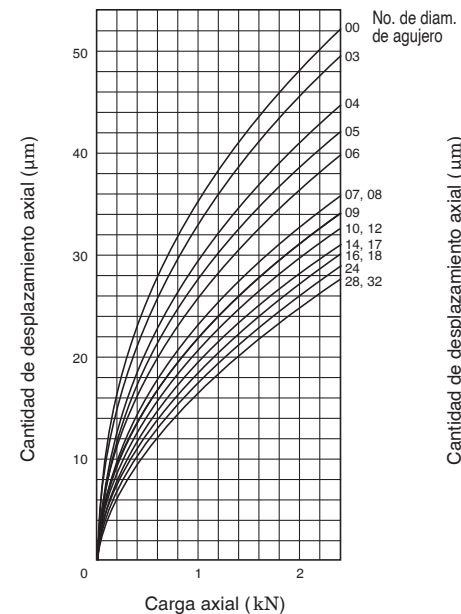
(1) 7900C (Ángulo de contacto)15°
