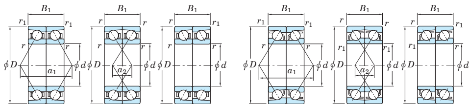
Espalda con espalda DB Cara con cara DF Tandem DT (Con jaula mecanizada)
