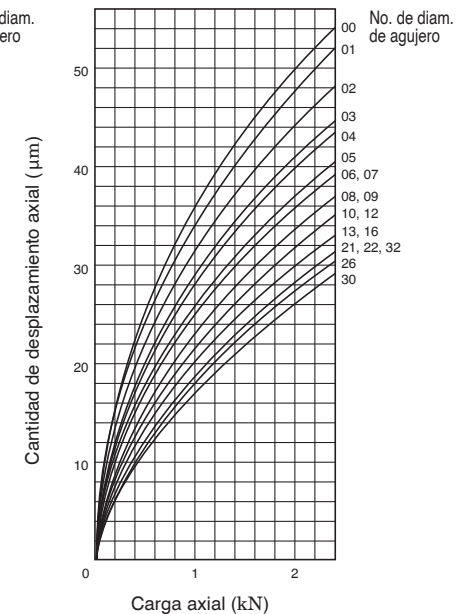
(2) 7000C (Ángulo de contacto)15°
