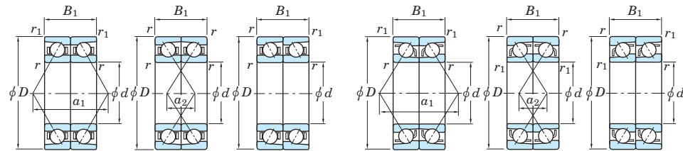
Espalda con espalda DB Cara con cara DF Tandem DT (Con jaula mecanizada) Espalda con espalda DB Cara con cara DF Tandem DT (Con jaula prensada)
