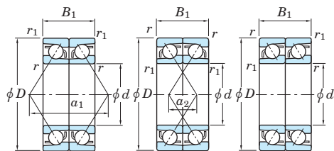
Espalda con espalda DB Cara con cara DF Tandem DT (Con jaula prensada)
