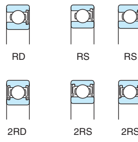
Sellos con contacto extremadamente ligero
